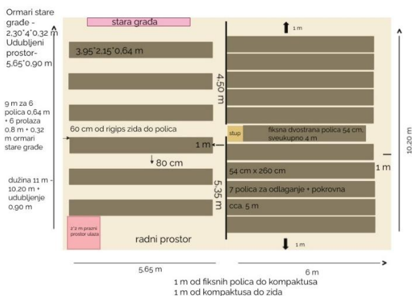
Slika 15. Radna skica opremanja spremišta djelomično s fiksnim policama, djelomično s kompaktusima
